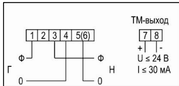
Рисунок В.9 – Схема включения счетчиков CE 102 тип корпуса S7, исполнения «JR1KVZ», «JKPVZ», «JKR1QVZ», «JKPQVZ»
