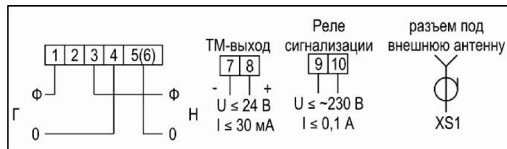
Рисунок В.6 – Схема включения счетчиков СЕ 102 тип корпуса S7, исполнения «OKR2SVZ», «OKQR2SVZ»
