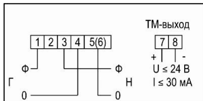
Рисунок В.23 – Схема включения счетчиков CE 102 тип корпуса R5, исполнения «ОК»
