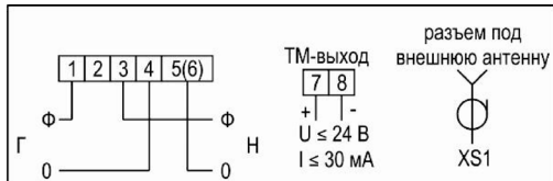
Рисунок В.5 – Схема включения счетчиков СЕ 102 тип корпуса S7, исполнения «JR2KVZ», «JKR2QVZ»
