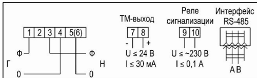
Рисунок В.3 – Схема включения счетчиков СЕ 102 тип корпуса S7, исполнения «AOKSVZ», «AOKQSVZ»
