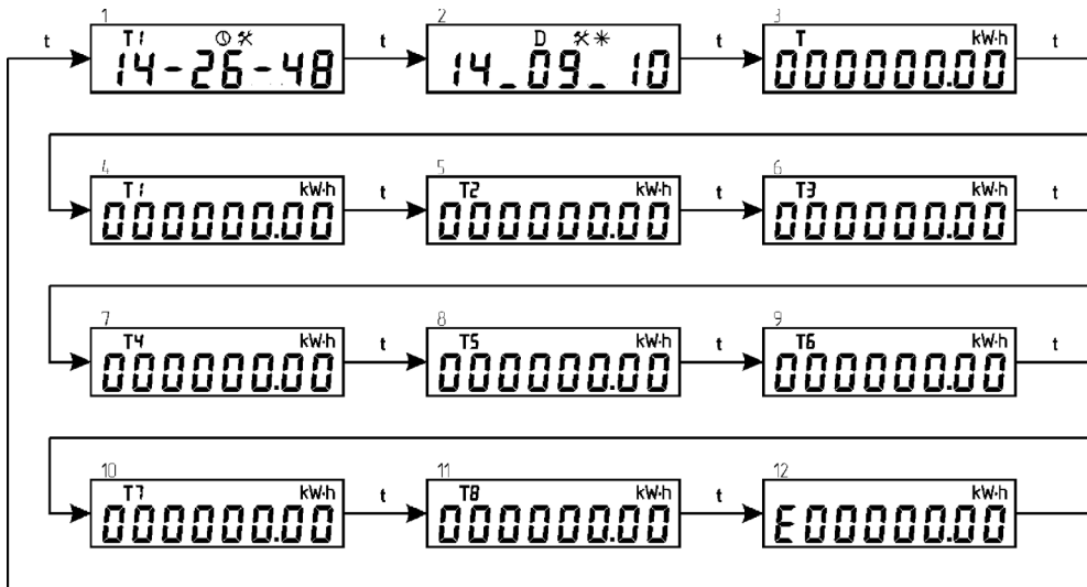
Рисунок 8.1 – Режим автоматической смены индикации счетчика
