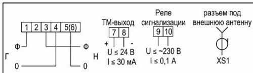
Рисунок В.7 – Схема включения счетчиков СЕ 102 тип корпуса S7, исполнения «JR2KSVZ»
