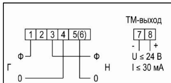
Рисунок В.8 – Схема включения счетчиков СЕ 102 тип корпуса S7, исполнения «OKPQVZ»
