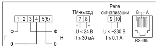
Рисунок В.4 – Схема включения счетчиков СЕ 102 тип корпуса S7, исполнения «JAKSVZ», «JAKQSVZ»
