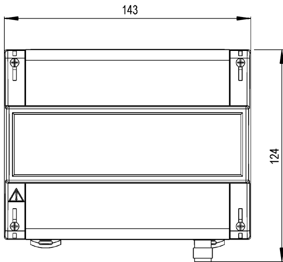
Рисунок Б.4 – Габаритные и установочные размеры счетчика CE 102 R8 (для исполнений «R2»)
