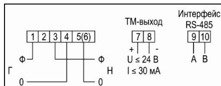
Рисунок В.24 – Схема включения счетчиков CE 102 тип корпуса R5, исполнения «АК»
